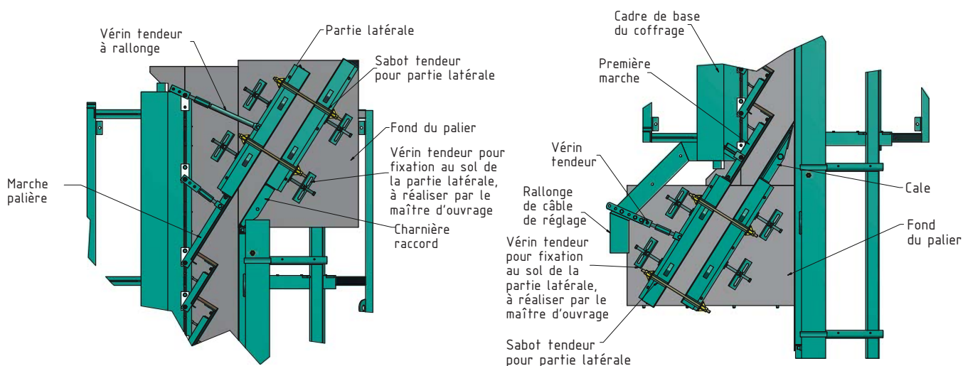
Palier pour fin de marches
